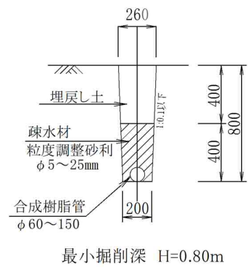
標準図（暗渠排水）
