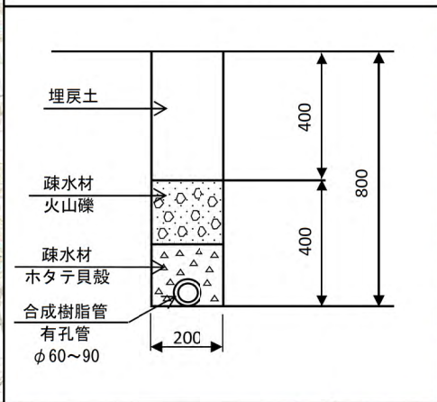
暗渠排水標準断面図
