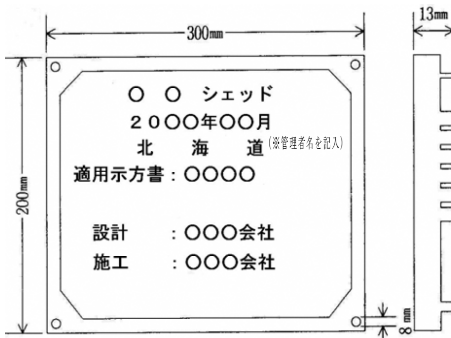
図8-1 履歴板
