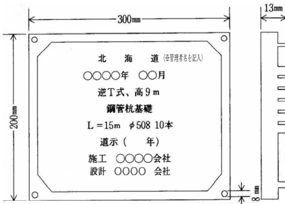
図3-1 橋歴板
